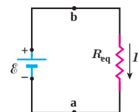
شکل ۲۰-۲ مدار معادل شکل ۱۹-۲ جریان آنها داریم: که در آن سه مقاومت با مقاومت R_{eq} جایگزین شده است.
